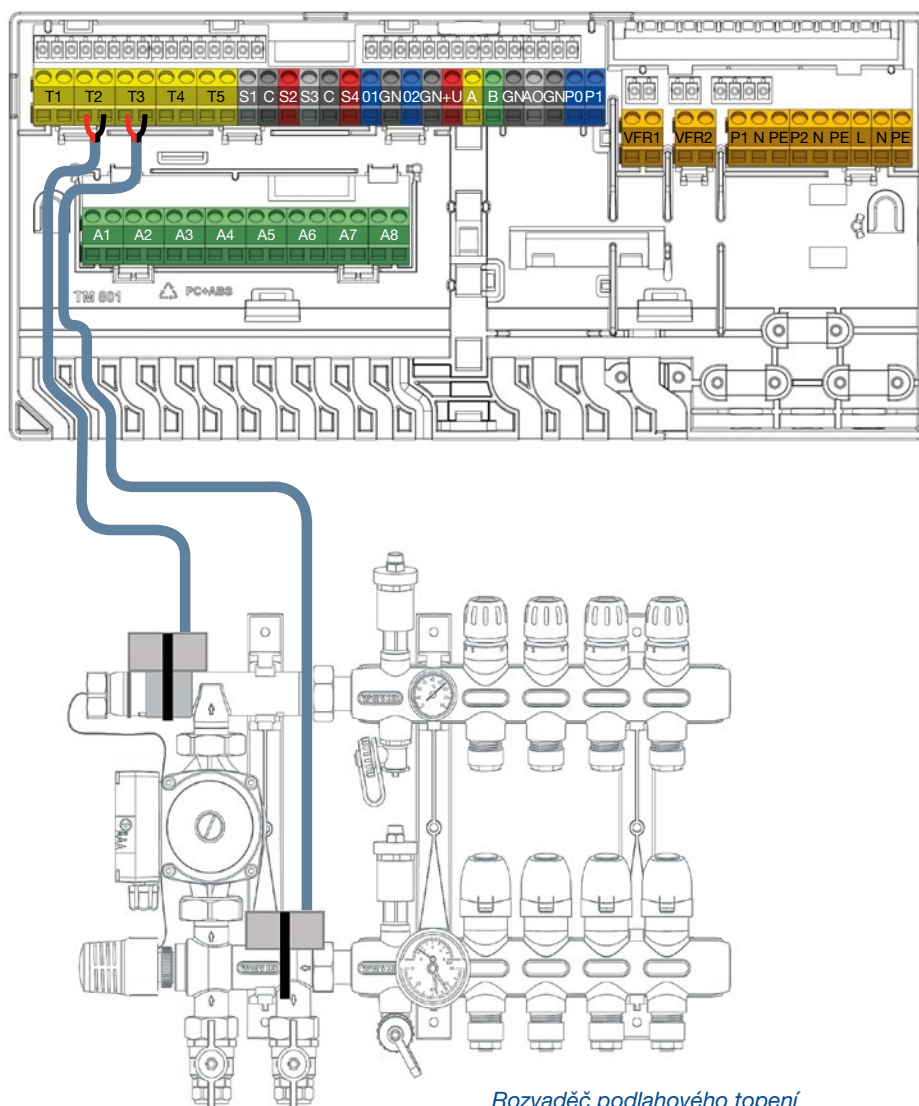
Rozvaděč podlahového topení
