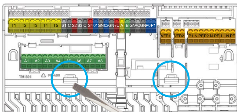
Demontáž CCU a EU z lišty DIN
