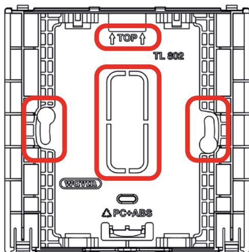
Zadní deska rámečku nástěnné krabice
