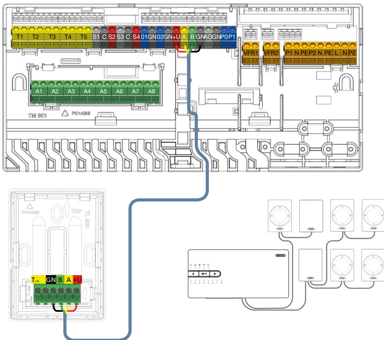
Připojení kabelových pokojových termostátů a senzorů prostřednictvím sběrnice kabelu
