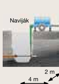
Koncový výkop během zatahování potrubí
