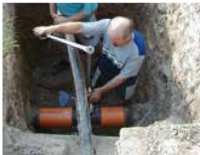
Vysazení přípojeky pomocí sedlové tvarovky
