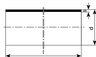
Dvouvrstvé potrubí PE 100 Vnějších 10 % barevně odlišeno.
