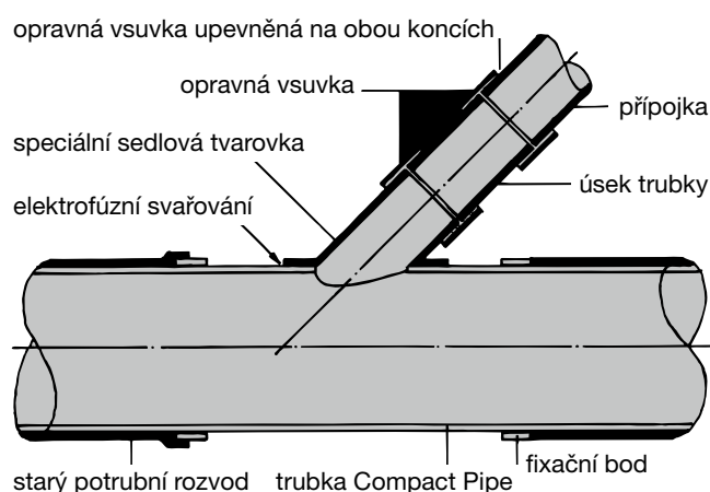
Vysazení odbočky v montážní jámě pomocí sedlové tvarovky
