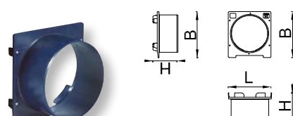
Šachtový adaptér 315 Q-Bic Plus
