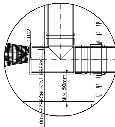
Šachta Tegra 1000 s regulačním prvkem DN 160 typ T – detail
