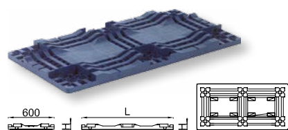
Dno uzavřené Q-Bic Plus
