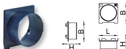
Vstupní deska DN 315 Q-Bic Plus
