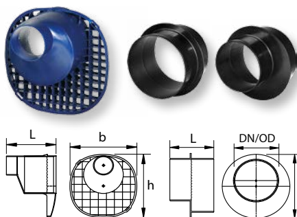
Vstupní hrdlo
