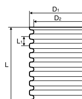
Zasakovací šachta Wavin – Tegra 425
