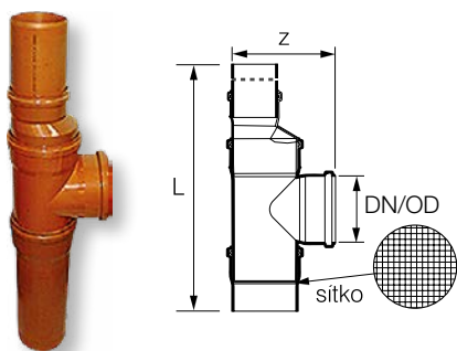
Filtr pro dešťovou šachtu
