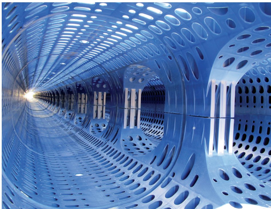
Wavin Q-bic z uceleného systému Intesio slouží k vytvoření retenčního prostoru pro objem náhrvového deště
