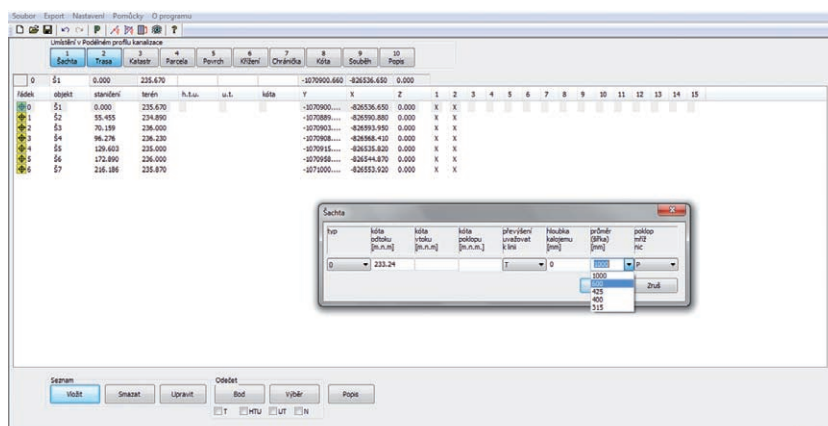
AutoPEN Wavin modul Situace pro odečet souřadnic trasy liniové stavby přímo ze situační mapy v prostředí AutoCAD
