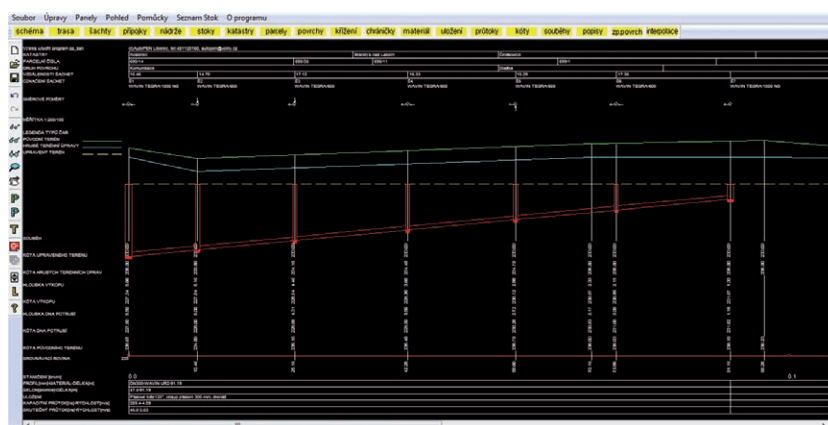
Modul Podélný profil kanalizace slouží k návrhu podélného profilu kanalizace a terénu
