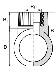
Navařovací sedlo s vnitřním závitem
