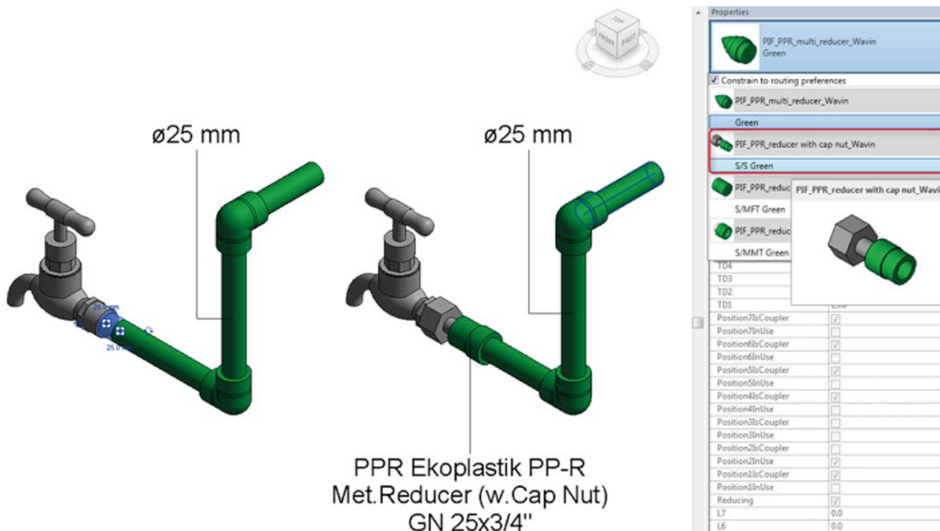
Ukázka řešení závitového přechodu s převlečnou maticí pro systém zadaný pomocí DN
