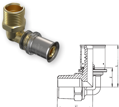
Wavin M5 – Koleno 90° – vnější závit
