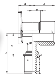
Wavin M1 (M-press) – Nástěnné koleno 90° – vnitřní závit prodloužený
