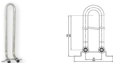
Radiátorová přípojka - do podlahy
