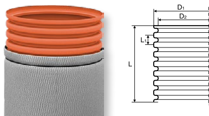
Zasakovací šachta Wavin – Tegra 1000 NG
