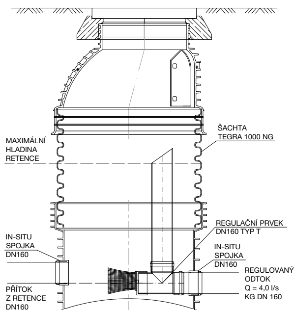
Šachta Tegra 1000 s regulačním prvkem DN 160 typ T – řez
