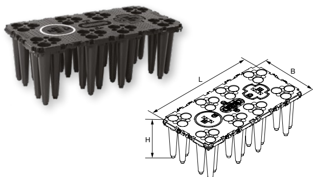
Akumulační box
