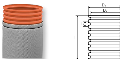
Zasakovací šachta Wavin – Tegra 600
