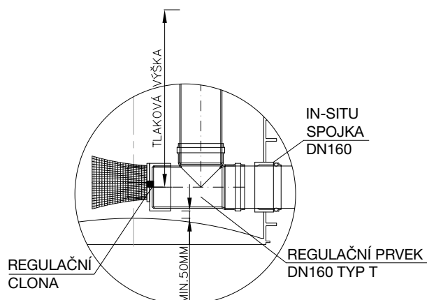
Šachta Tegra 1000 s regulačním prvkem DN 160 typ T – detail
