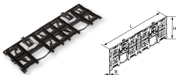
Boční deska
