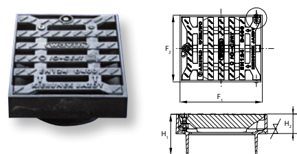
Litinová mříž D400 Ø 315 mm – do teleskopické roury
