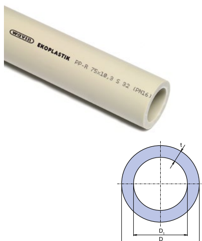
Trubka Ekoplastik PPR S 3,2 / PN 16 / SDR 7,4
