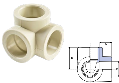
Koleno trojcestné
