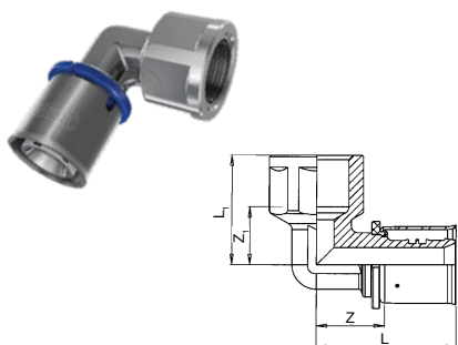
Wavin M1 (M-press) – Koleno 90° – vnitřní závit
