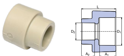
Redukce hrdlová
