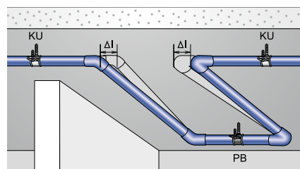
U-kompenzátor
