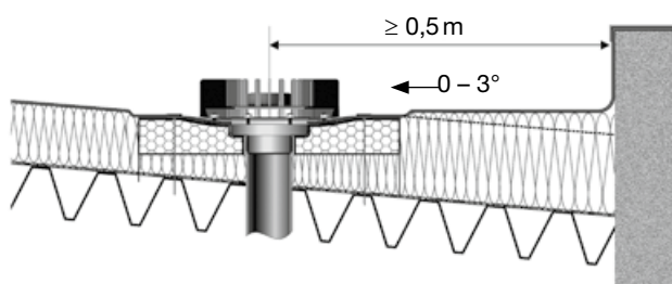
Umístění a okolí střešního vtoku
