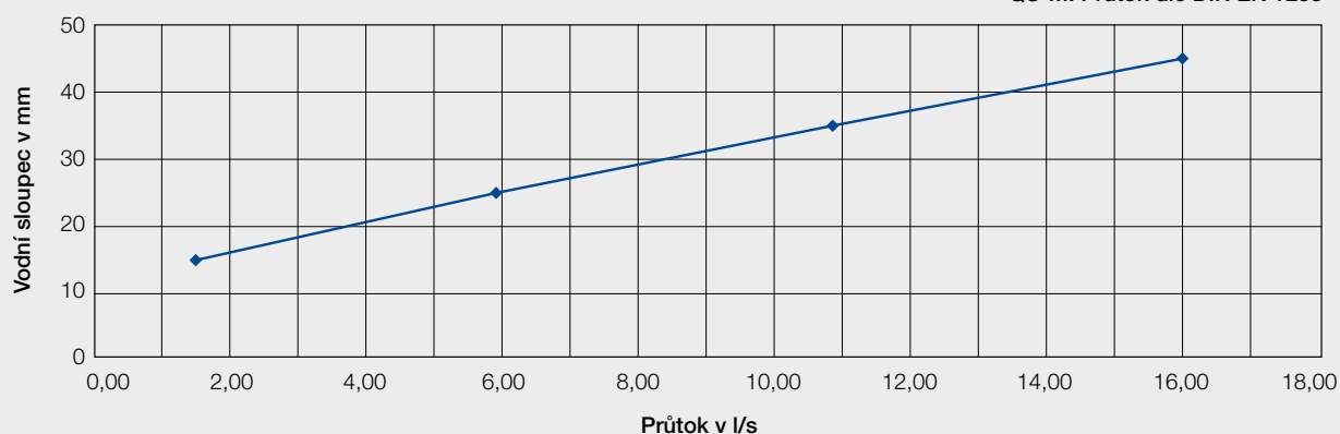
Kapacitní křivka QS-M fóliový typ
