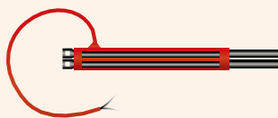
Elektrické vyhřívání 230 V/10 W
