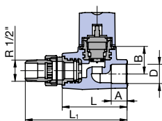
Radiátorový termostatický ventil přímý
