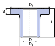
Lemový nákrůžek
