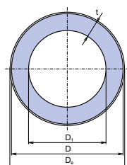
Trubka Ekoplastik Stabi Plus S 4 / SDR 9 PN 22 (výpočet) s perforovanou fólií
