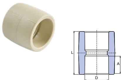
Nátrubek
