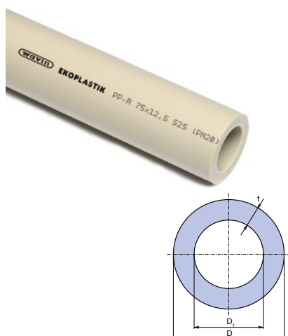
Trubka Ekoplastik PPR S 2,5 / PN 20 / SDR 6
