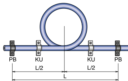
Uskočení U-kompenzátoru pod trasu potrubí
