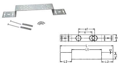
Držák nástěnných kolien
