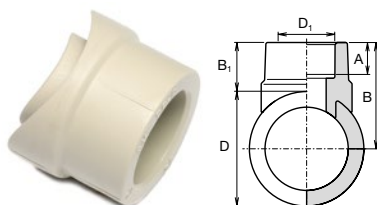
Navařovací sedlo
