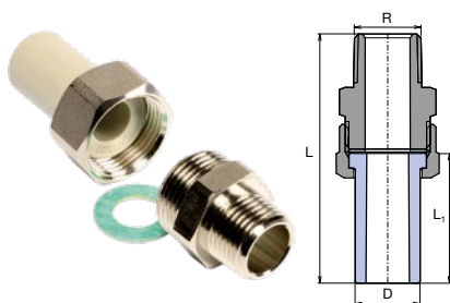
Šroubení vnější
