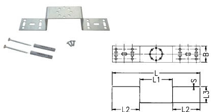
Držák nástěnného kolena
