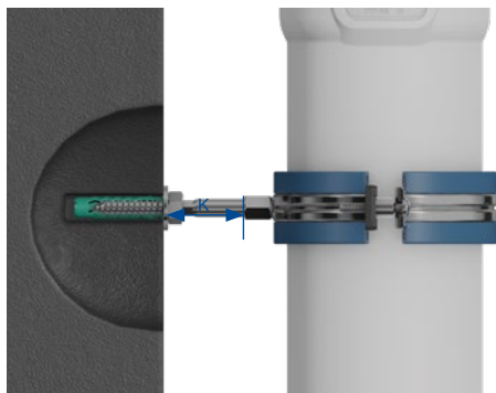
Max. délka závitové tyče
