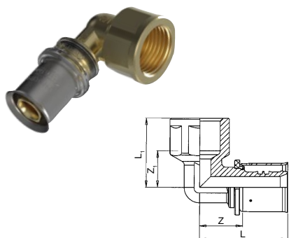
Wavin M5 – Koleno 90° – vnitřní závit
