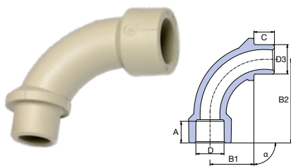
Oblouk
